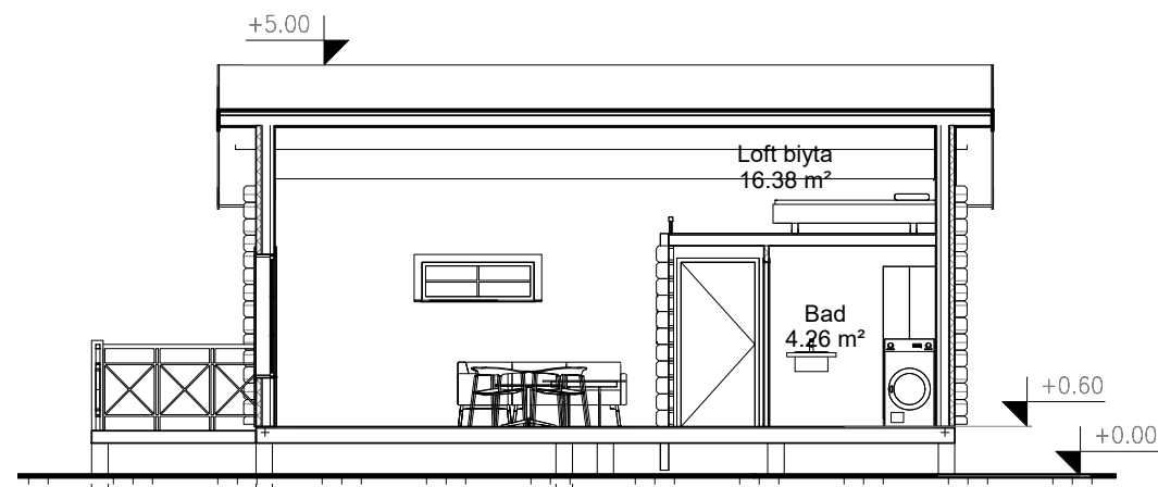
1 Sektion 2 1 : 100
