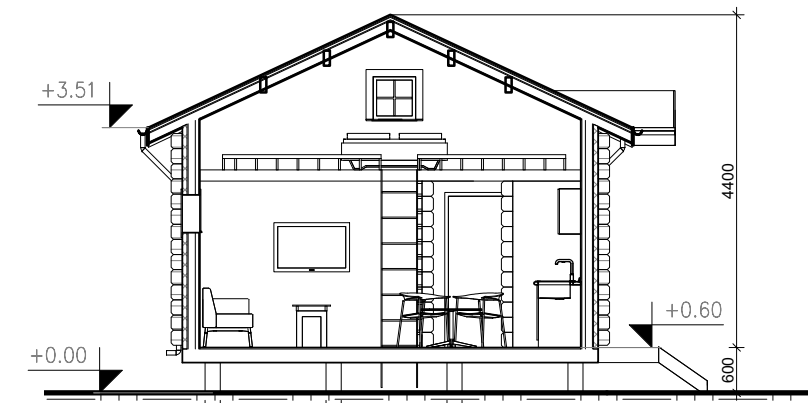
2 Sektion 1 1 : 100
