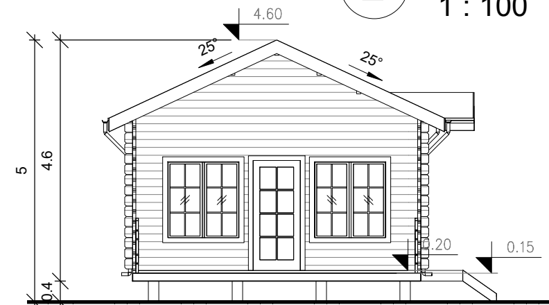
4 Fasad 4 1 : 100
