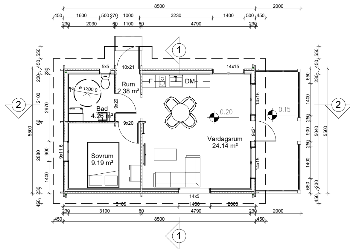
1 Marknivå 1 : 100
