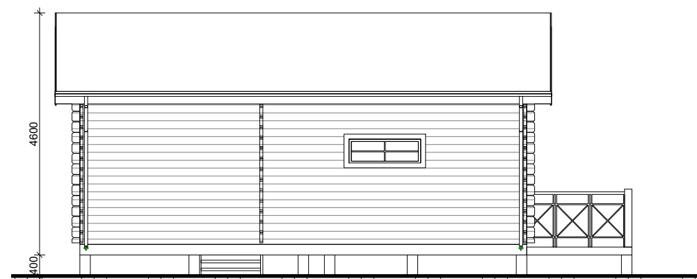
3 Fasad 1 1 : 100
